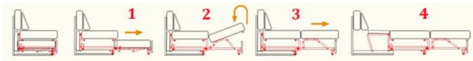
Принцип работы механизма ТТ
